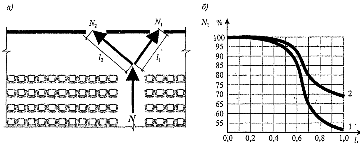
а – схема распределения потока численностью N , чел.; б – влияние соотношения между расстояниями до выходов на распределение численности людей из общего потока, направляющихся: 1 – к ближайшему из двух одинаковых выходов l_1 : наружу, в лестничные клетки, на открытые лестницы; 2 – к открытой лестнице l_1 или в лестничную клетку l_2
